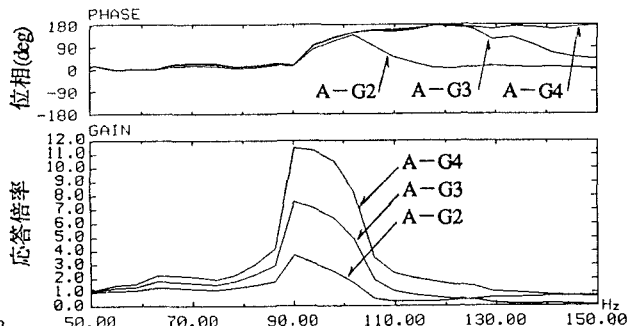
図4 地盤の各深度の周波数伝達関数 (エルセントロ波NS成分入力)
