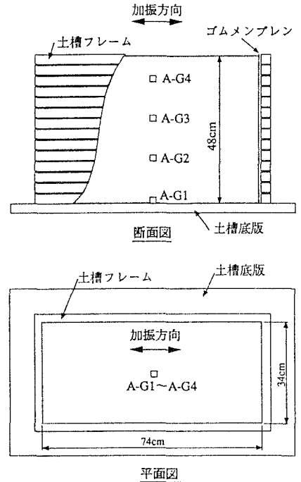
図1 せん断土槽外観および計器配置
