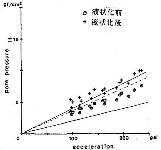
図2 加振時の間隙水圧振幅 (H = 20cm)
