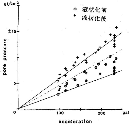
図3 加振時の間隙水圧振幅 (H = 30cm)
