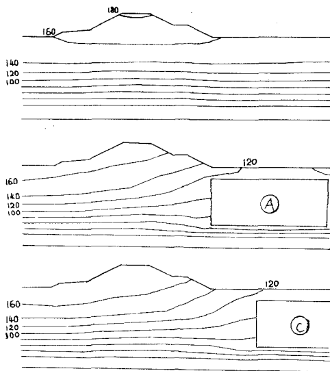
図-6 変位応答の分布 ( 10^{-2} cm)
