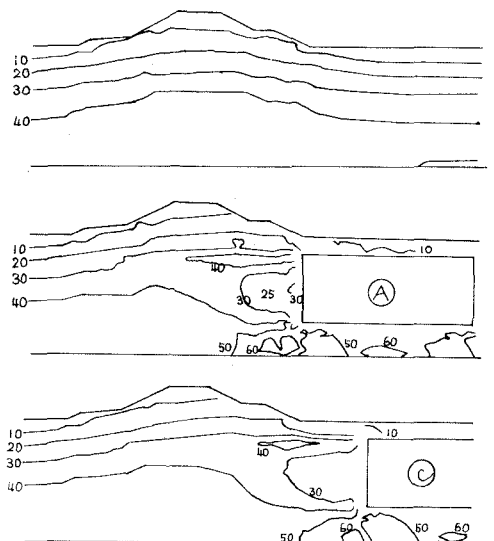
図-7 セン断応力の分布 ( 10^{-2} Kg/cm 2 )
