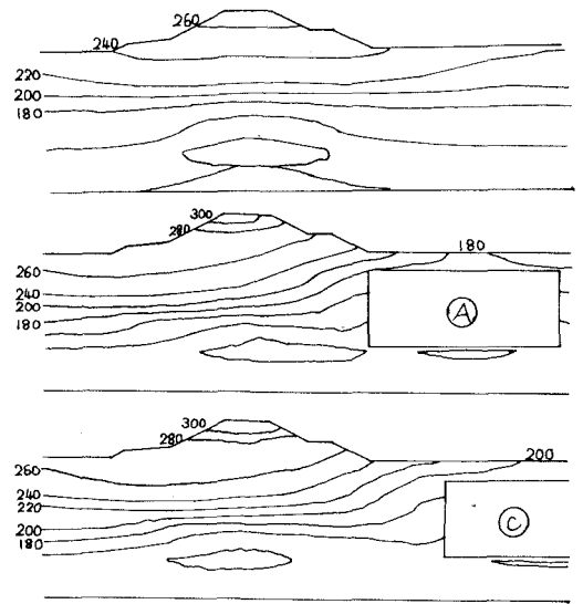
図-5 加速度応答の分布 (gal)
