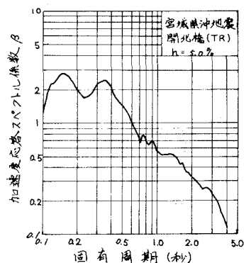
図-3 入力地震動の加速度応答スペクトル
