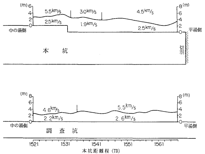
図-4 地山速度、ゆるみ領域の解析結果
