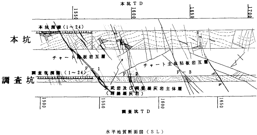
水平地質断面図 (S L) 図-6 試験区間の地質構造
