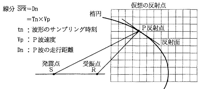
図-5 反射面の位置と分布
