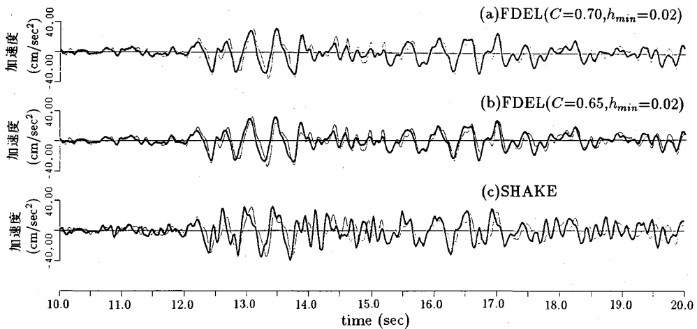
図一 地中 (G.L. -38.5 m) での推定値と観測記録の比較 (新大田観測点, 千葉県東方沖地震, 太い実線が計算値, 細い実線が観測記録)
