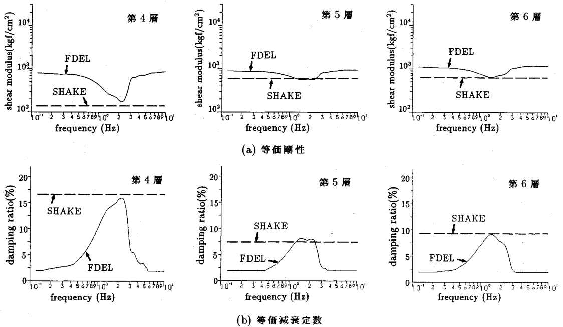
図-8 地盤各層における等価剛性, 等価減衰定数 (表-1 の新大田観測点の層番号に対応, (千葉県東方沖地震, comp. = N 095 E))
