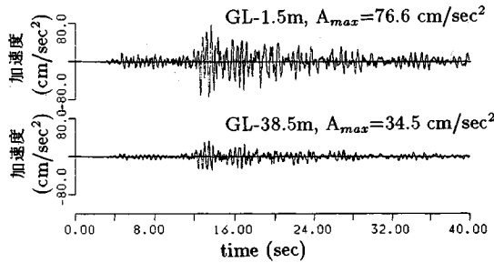
図-5 新大田アレー観測点での地震動記録 (千葉県東方沖地震, comp. = N 095 E)
