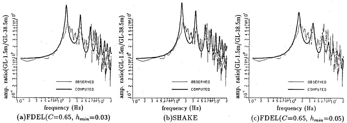
図-10 本手法 (FDEL) および SHAKE による推定値と観測記録における増幅特性の比較 (新大田観測点, 南関東東方沖地震, comp. = N 095 E)
