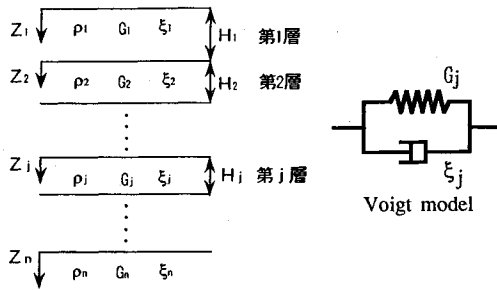
図一 多層地盤モデル
