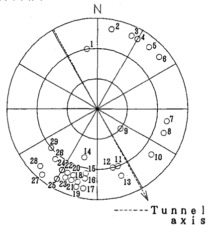
図-4 シュミットネットに示す割れ目およびトンネル軸
