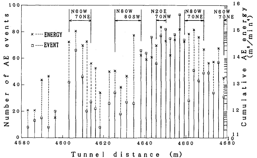
図-6 切羽あたりのAE発生数ならびに累積エネルギーの推移状況
