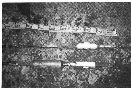
写真-1 発振(下)・受振装置(上)
