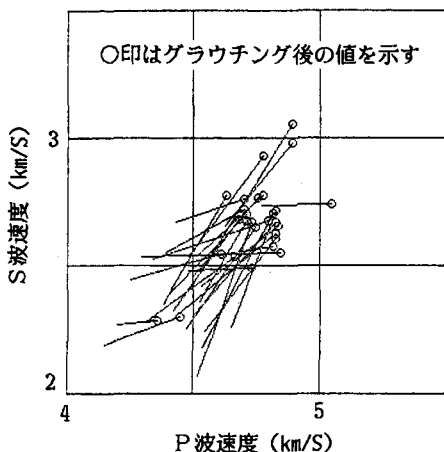
図-9 P波・S波速度の相関変化
