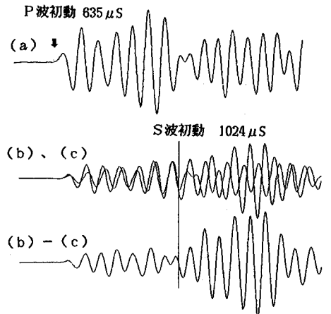
図-5 P波・S波の読み取り例
