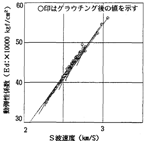
図-13 S波速度と動弾性係数の相関変化
