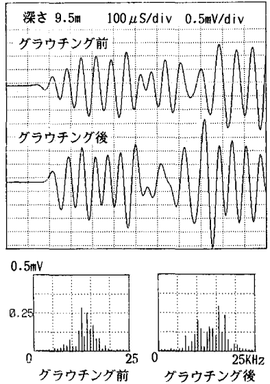
図-4 波形例、周波数スペクトル
