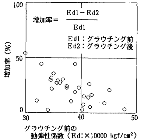
図-11 動弾性係数の変化
