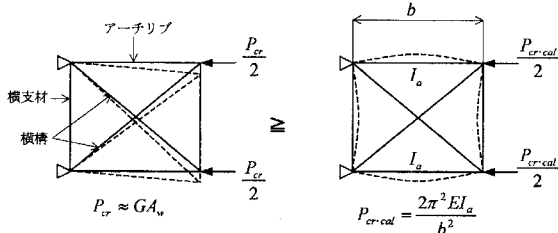
(a) パネル間のせん断座屈
