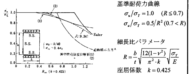
図 8.13 3辺単純1辺自由の圧縮版の臨界応力度曲線 (17)
