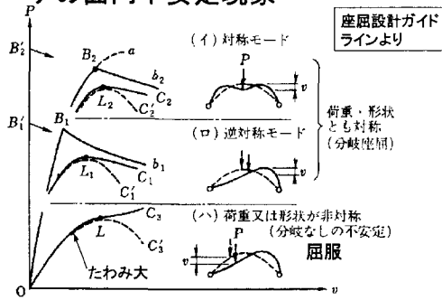
図 12.1 アーチ面内不安定における荷重-面内たわみ関係
