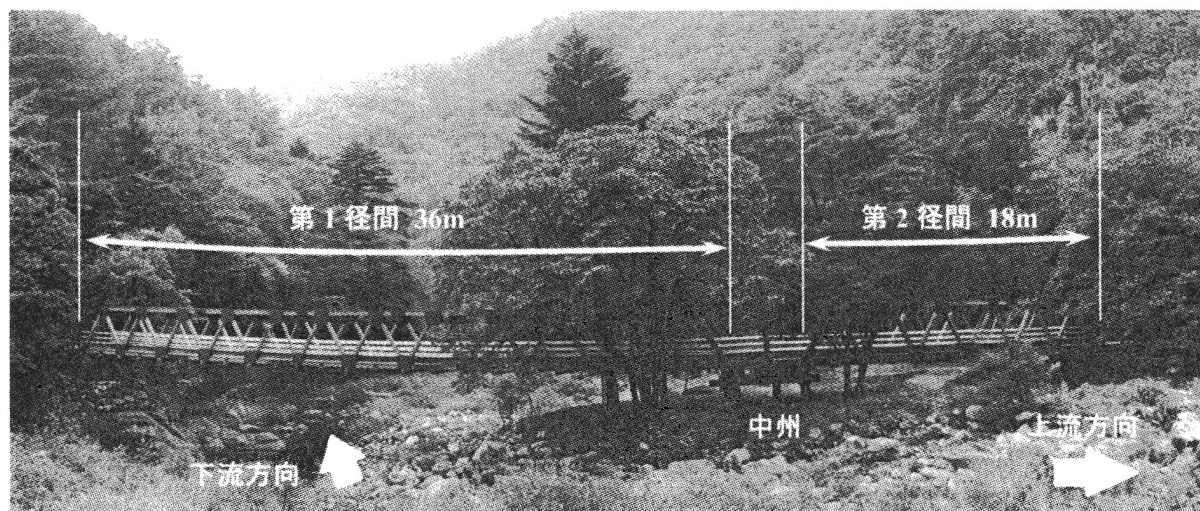
写真1 対象橋梁の全景(2003/11/06 撮影・4枚を合成)
