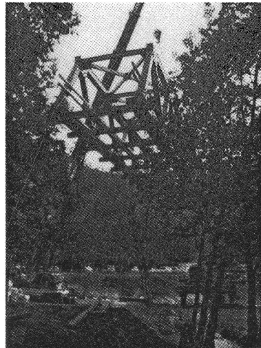
写真4 2回目往路 架橋原位置から吊上げ 16:22:02
