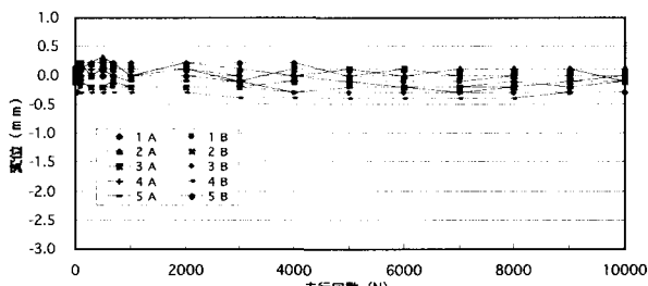
図-22 コンクリート舗装の目地段差の変化
