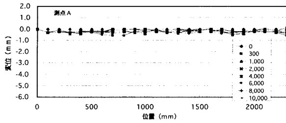
図-11 PC床版舗装のわだち形状
