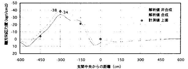
図-18 PC床版試験体の舗装上面軸方向応力
