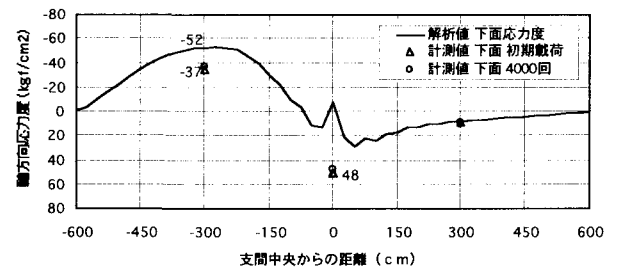
図-24 コンクリート舗装試験体のデッキプレート応力
