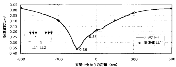
図-8 アスファルト舗装試験体のデッキプレートたわみ
