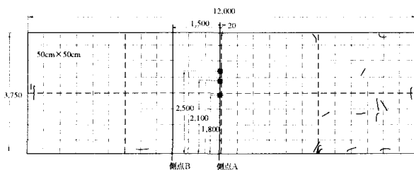
図-21 コンクリート舗装表面のクラック分布
