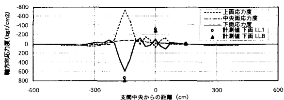
図-9 アスファルト舗装試験体のデッキプレート軸方向応力
