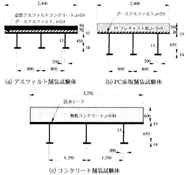
図-1 試験体の断面図
