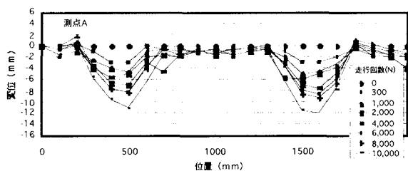
図-4 アスファルト舗装のわだち形状
