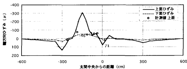
図-10 アスファルト舗装試験体の舗装軸方向ひずみ
