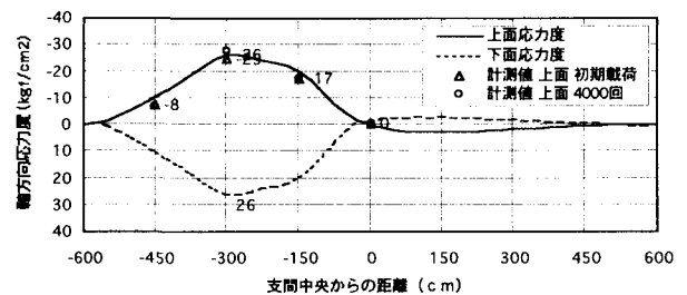
図-26 コンクリート舗装の軸方向応力
