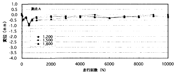
図-12 PC床版舗装のわだち変化
