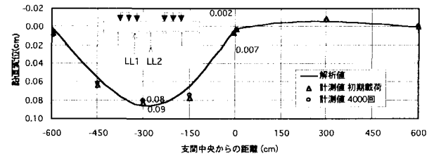
図-24 コンクリート舗装試験体のデッキプレートたわみ
