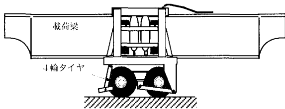
図-3 自動走行載荷装置
