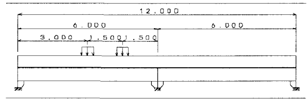
図-23 コンクリート舗装試験体の荷重位置
