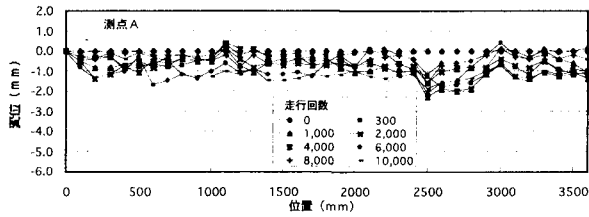
図-19 コンクリート舗装試験体のわだち形状
