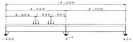
図-15 PC床版舗装試験体の荷重位置
