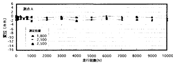
図-20 コンクリート舗装試験体のわだち形状
