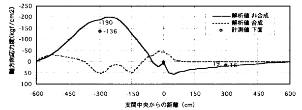
図-17 PC床版試験体のデッキプレート軸方向応力
