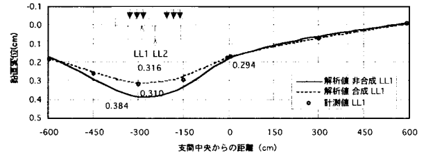
図-16 PC床版試験体のデッキプレートたわみ
