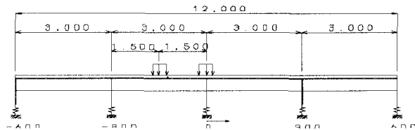
図-7 アスファルト舗装試験体の荷荷位置
