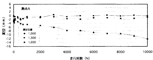
図-5 アスファルト舗装のわだち変化
