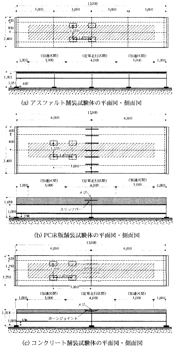
図-2 試験体の平面図、側面図
