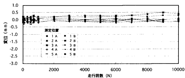
図-14 PC床版舗装の目地段差変化
