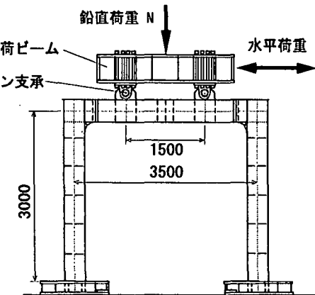
図-8 鋼ラーメン橋脚実験装置の概要 3)
