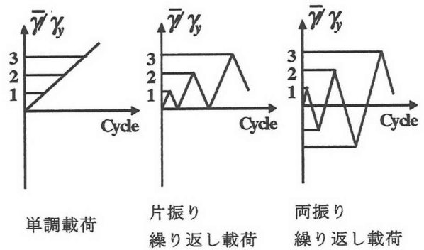
図-3 載荷方法
