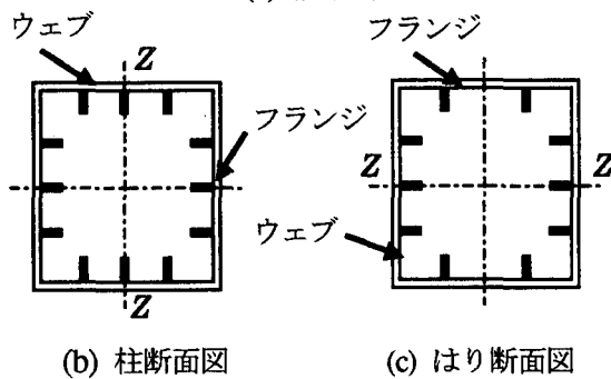
図-12 1層鋼製ラーメン橋脚
