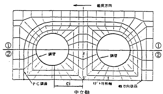
図-11 鋼管の応答分布
