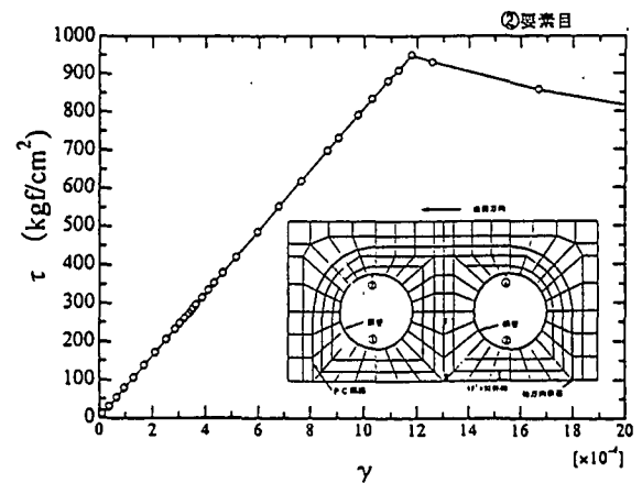
鋼管のせん断応力-せん断ひずみ関係
