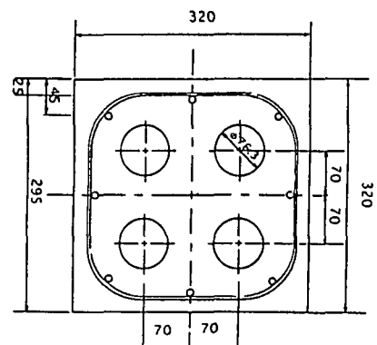
図-3 断面図
