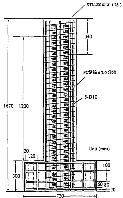
図-2 載荷実験供試体
