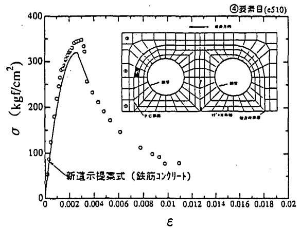
図-12 コンクリートの応力-ひずみ関係
