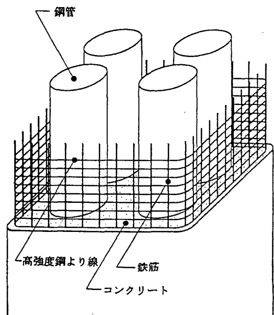
図-1 鋼管・コンクリート複合構造
