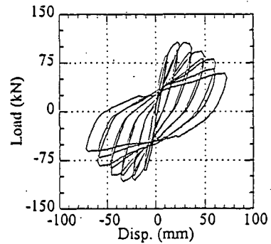
図-5 実験結果 (変位-荷重曲線)
