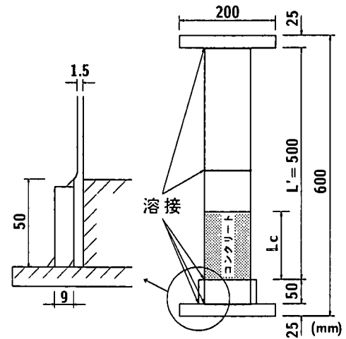
図-1 試験体の形状および寸法
