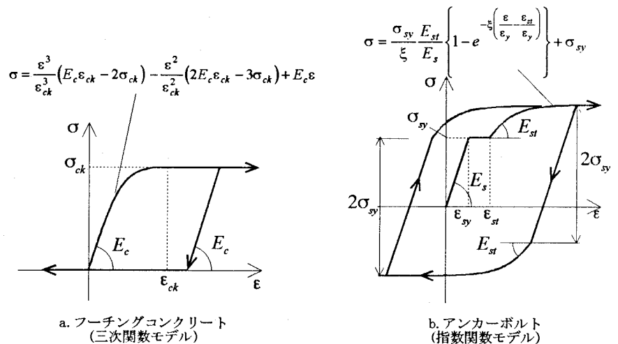
図 3.5.5 材料の応力-ひずみ関係
