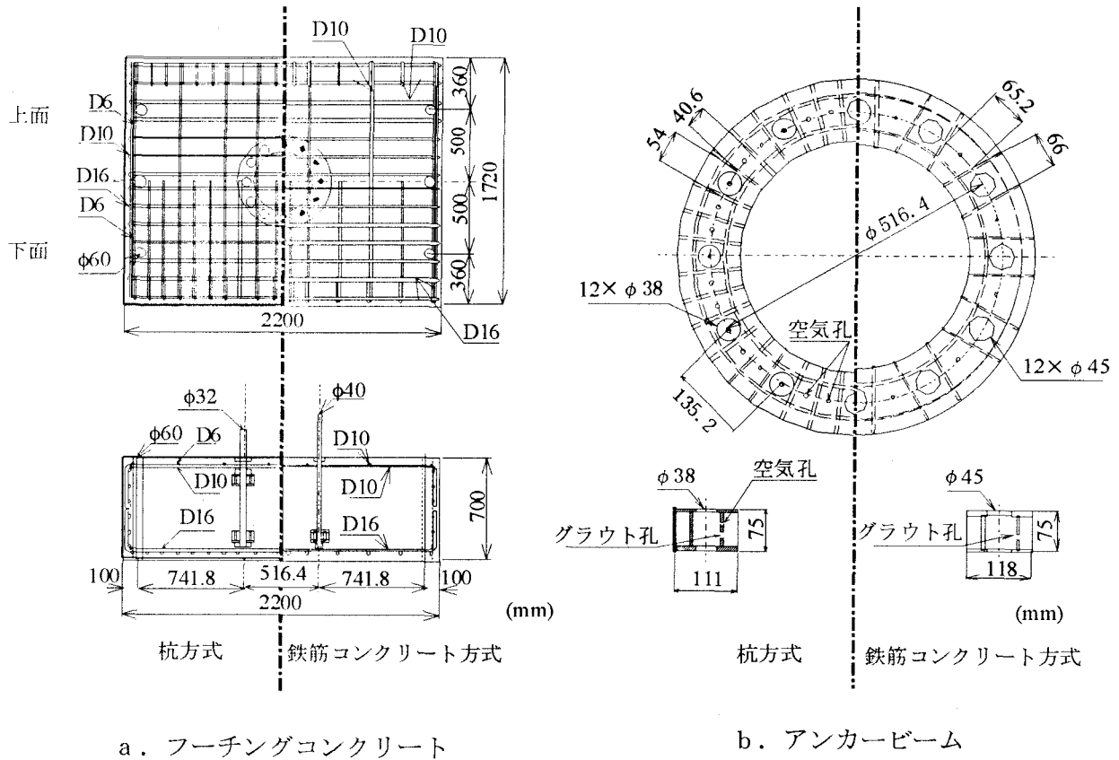
図 3.5.7 供試体形状
