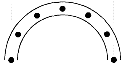
図 3.5.10 アンカーボルトの軸力分布 (杭方式)
