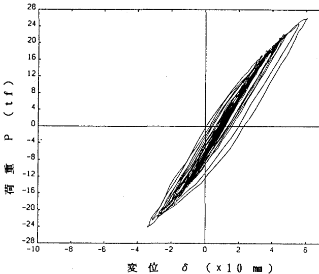
図-3.22 9シリーズ目のP～ \delta 曲線
