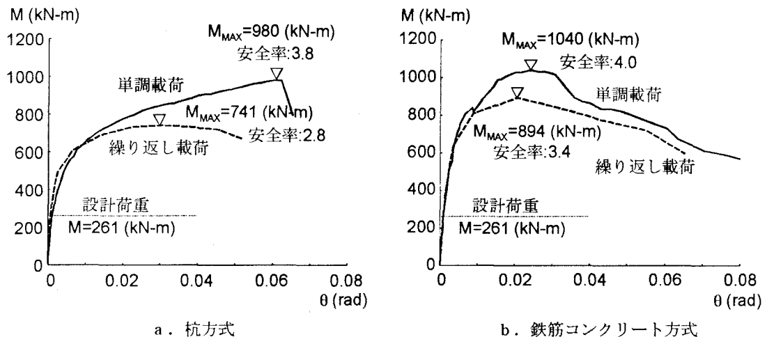
図 3.5.17 定着部の M- \theta 関係
