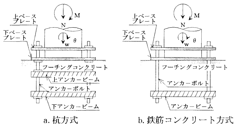
図-3.5.1 定着方式
