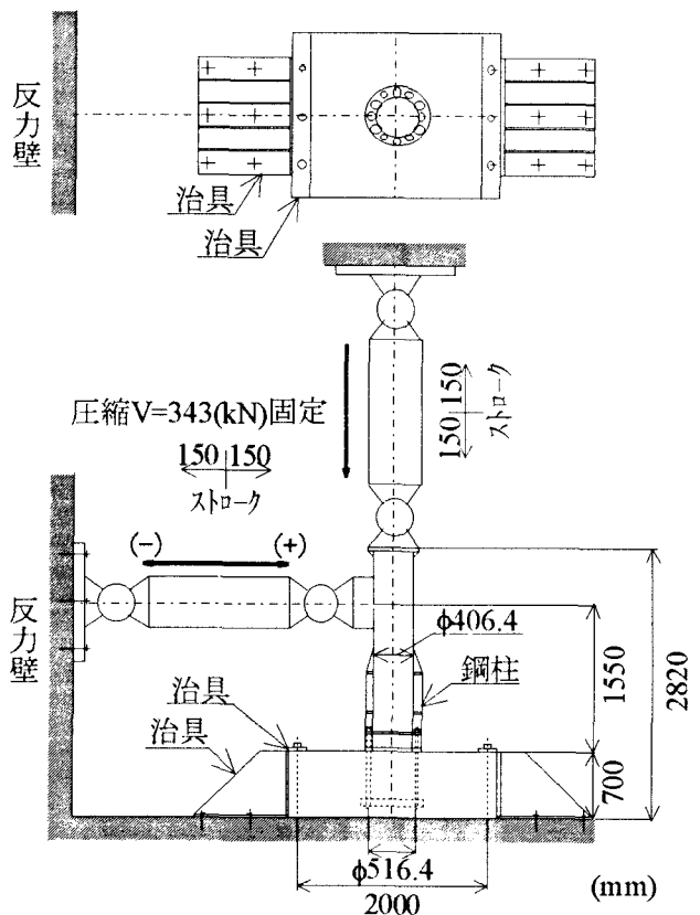
図 3.5.8 荷荷方法
