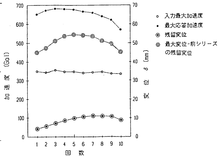
図-3.23 各シリーズ毎の加速度と変位
