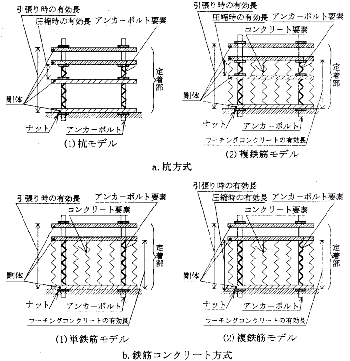
図 3.5.4 力学モデル
