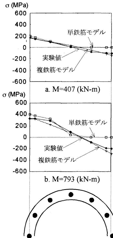
図 3.5.13 アンカーボルトの軸力分布 (鉄筋コンクリート方式)
