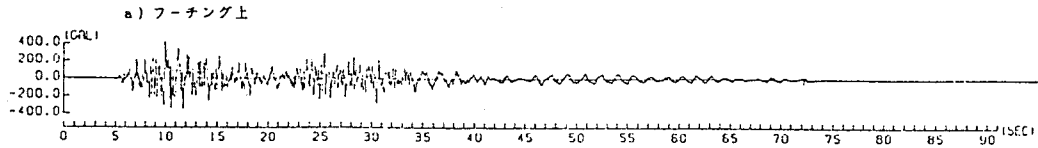
図 - 3.14 八郎瀉記録 4 倍入力 (最大応答加速度 432gal)
