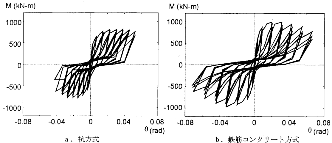
図 3.5.16 繰返し載荷時の M- \theta 関係
