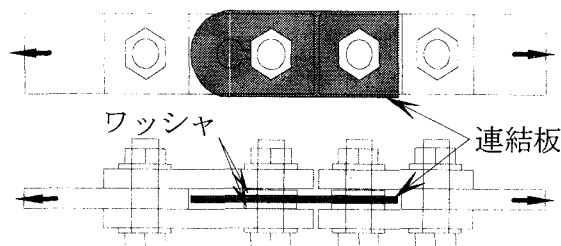
図 3.6.3 静的載荷用治具
