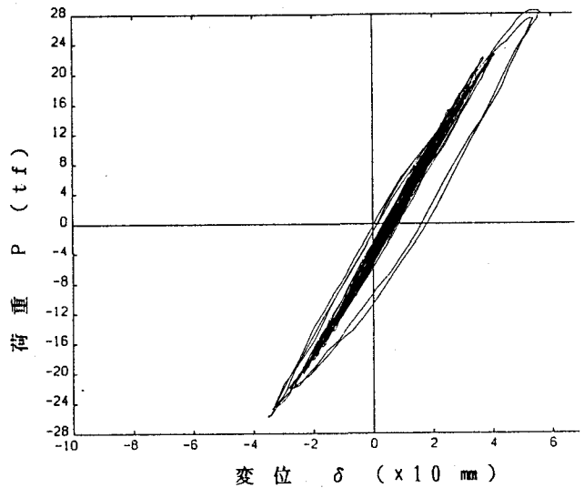
図-3.21 3シリーズ目のP～ \delta 曲線
