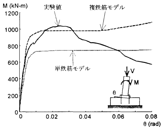
図 3.5.12 定着部の M-θ 関係 (鉄筋コンクリート方式)
