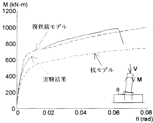
図 3.5.9 定着部の M-θ 関係 (杭方式)
