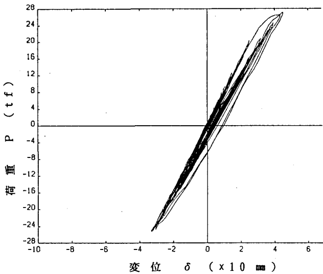
図-3.20 1シリーズ目のP～ \delta 曲線
