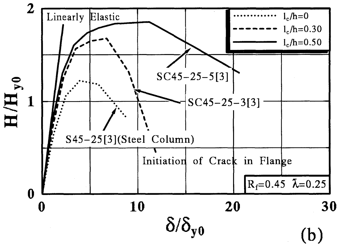
図 - 3.10 鋼柱とコンクリート充填柱の比較
