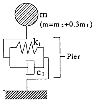
(a) 1 自由度系モデル
