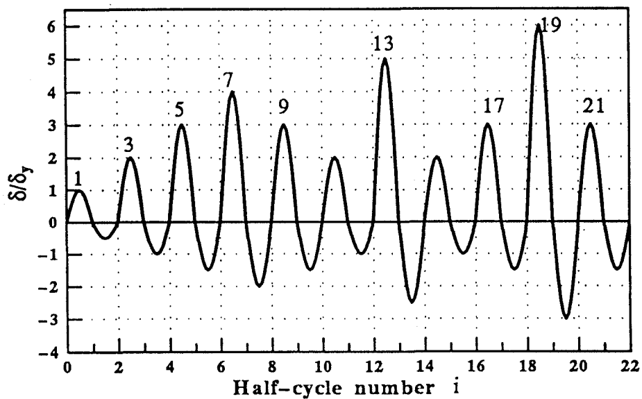
図4.6 想定応答変位図
