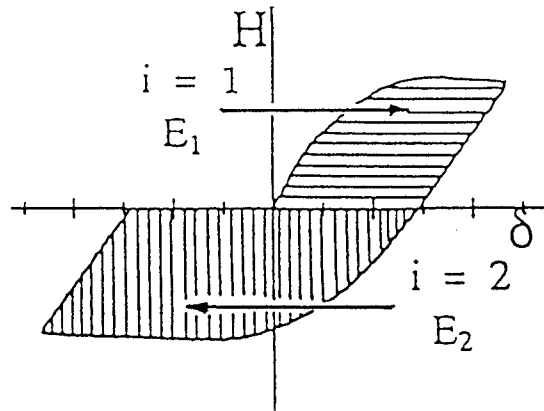
図 4.5 半サイクルのエネルギー吸収（消散量）
