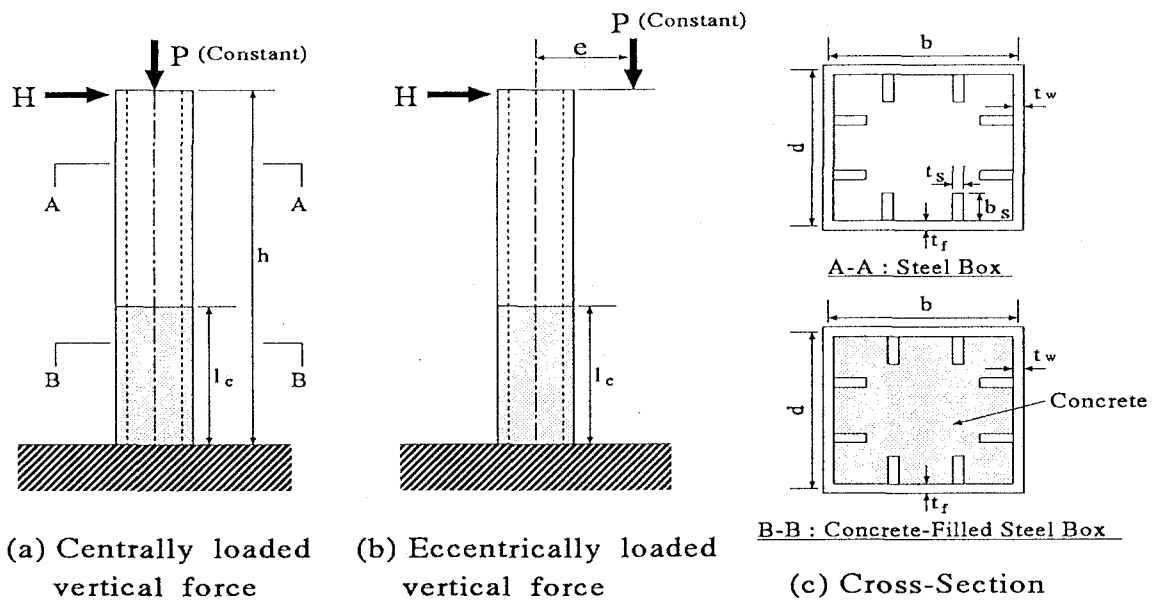
図 5.1.1 解析モデル
