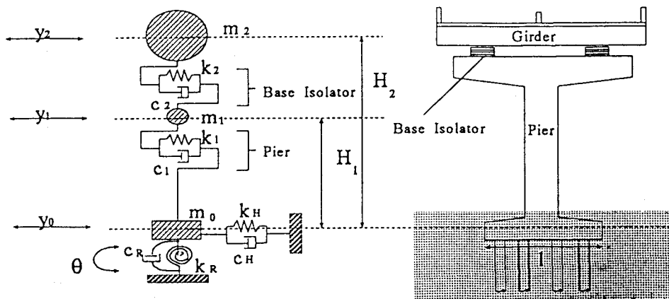
(c) 4 自由度系モデル
