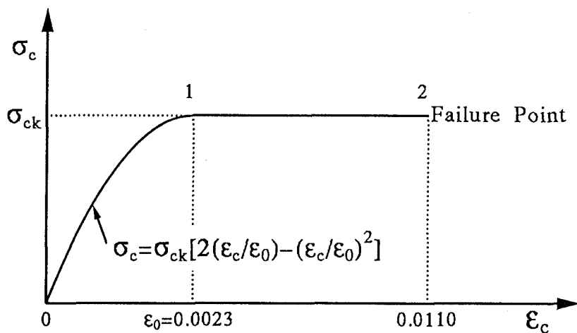
図 5.1.3 コンクリートの応力-ひずみ関係（圧縮）
