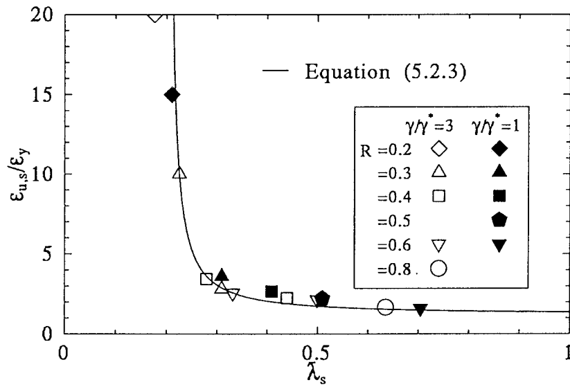
図 5.2.3 極限ひずみ \epsilon_{u,s} と \lambda_s の関係
