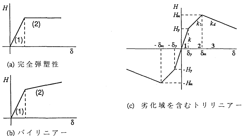
図 4.4 H- \delta 履歴曲線のスケルトンカーブ
