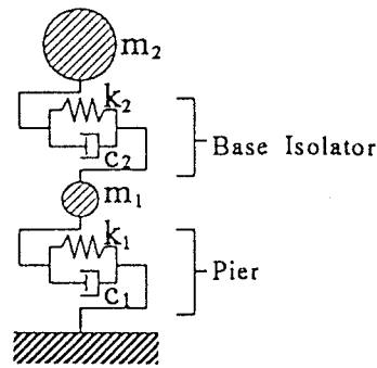
(b) 2 自由度系モデル
